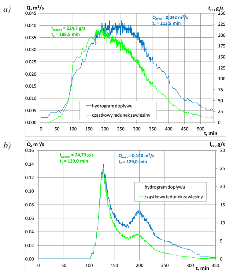
Rys. 3. Hydrogram dopływu Q=f(t) oraz krzywa opisująca zmienność ładunku zawiesiny ogólnej ( I_{cz.} ) w jednostce czasu ( dt ) dla wezbrania z dnia: a) 23.02.2010 r., b) 31.05.2010 r.
