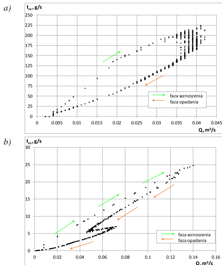
Rys. 5. Pętla histerezy zmian ładunku zawiesiny ogólnej ( l_{cz.} ) w funkcji przepływu ( Q ) dla wezbrania z dnia: a) 23.02.2010 r., b) 31.05.2010 r.
