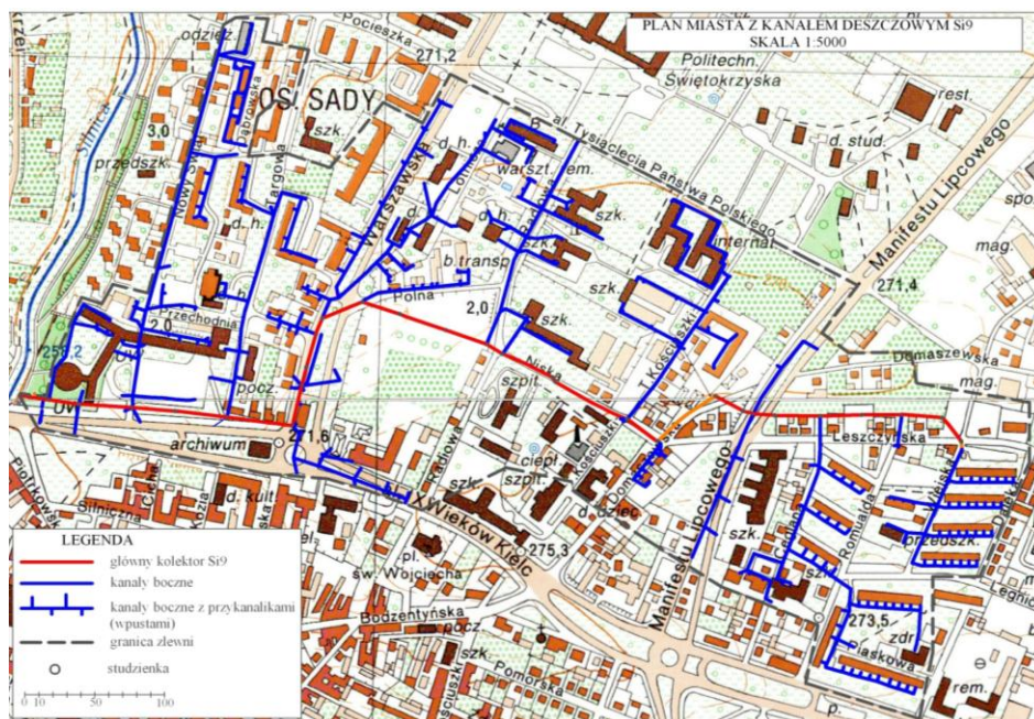
Rys. 1. Zlewnia kolektora Si9 wraz z układem kanałów bocznych [Dąbkowski i in. 2010] Fig. 1. Si9 collector catchment together with a system of lateral Canals [Dąbkowski et al. 2010]
